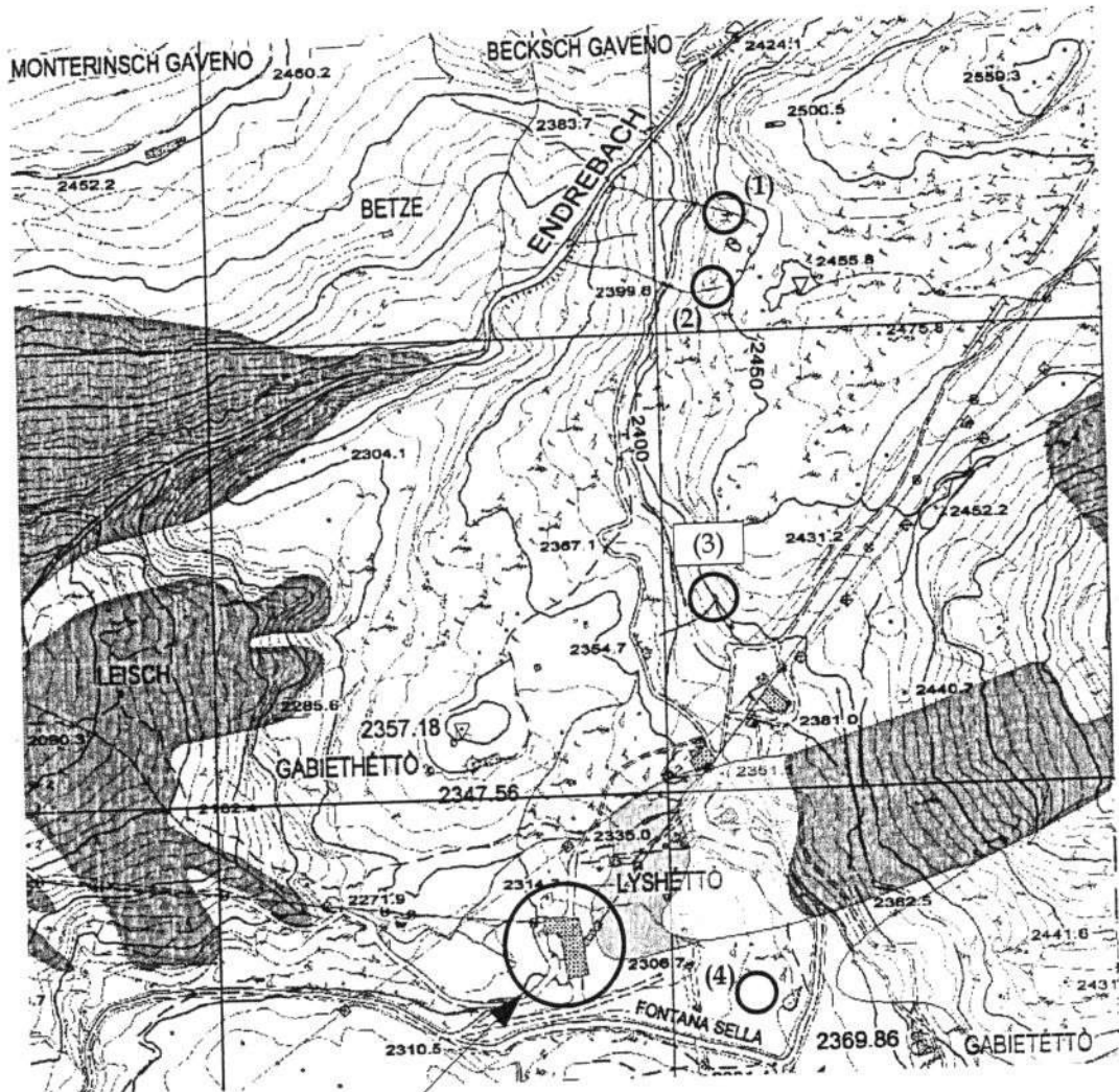
Opera di captazione "Fontana Sella", e vasca comunale del Gabiet.
